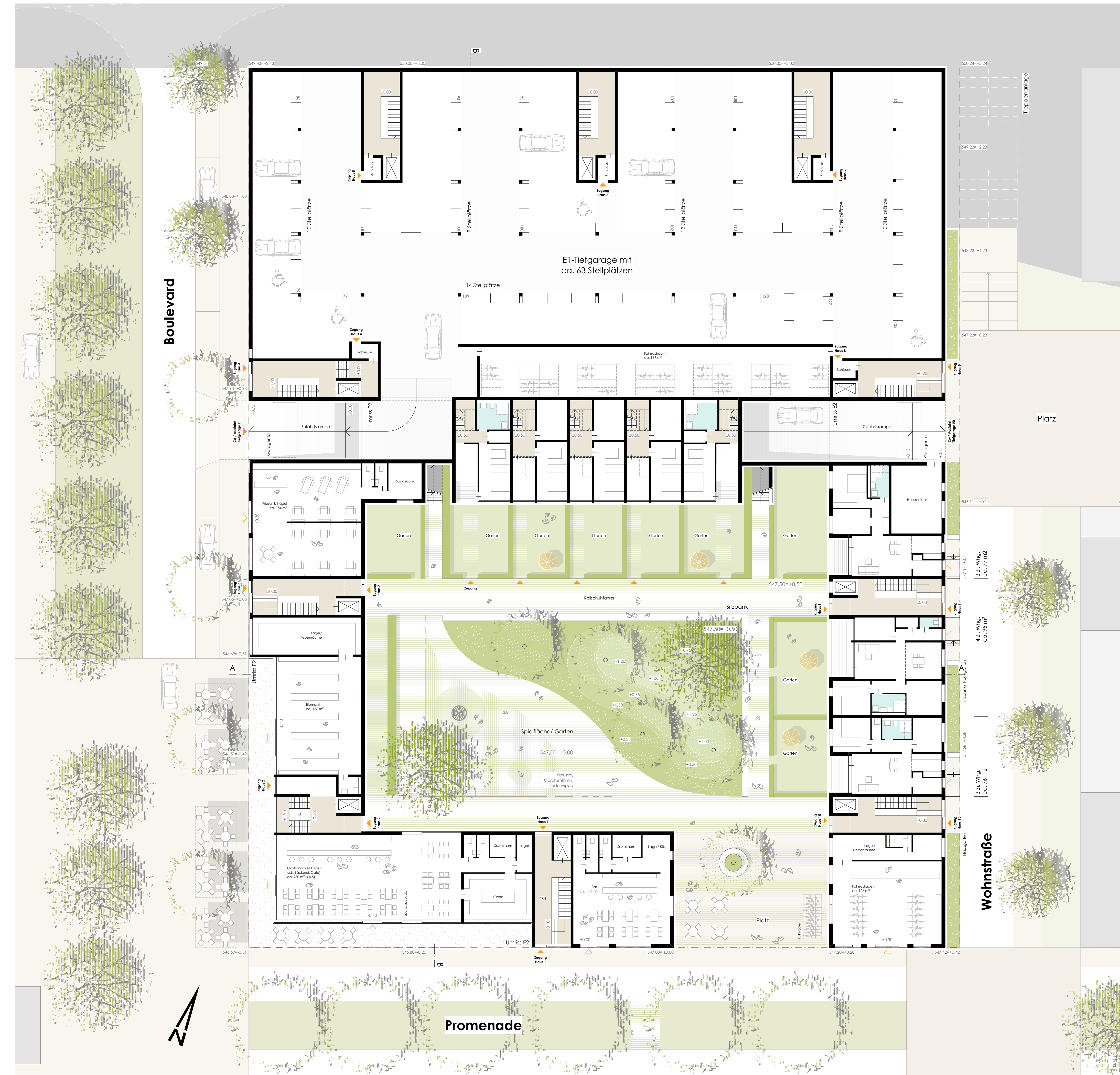
Ebene 1 (±0,00), M 1:200
