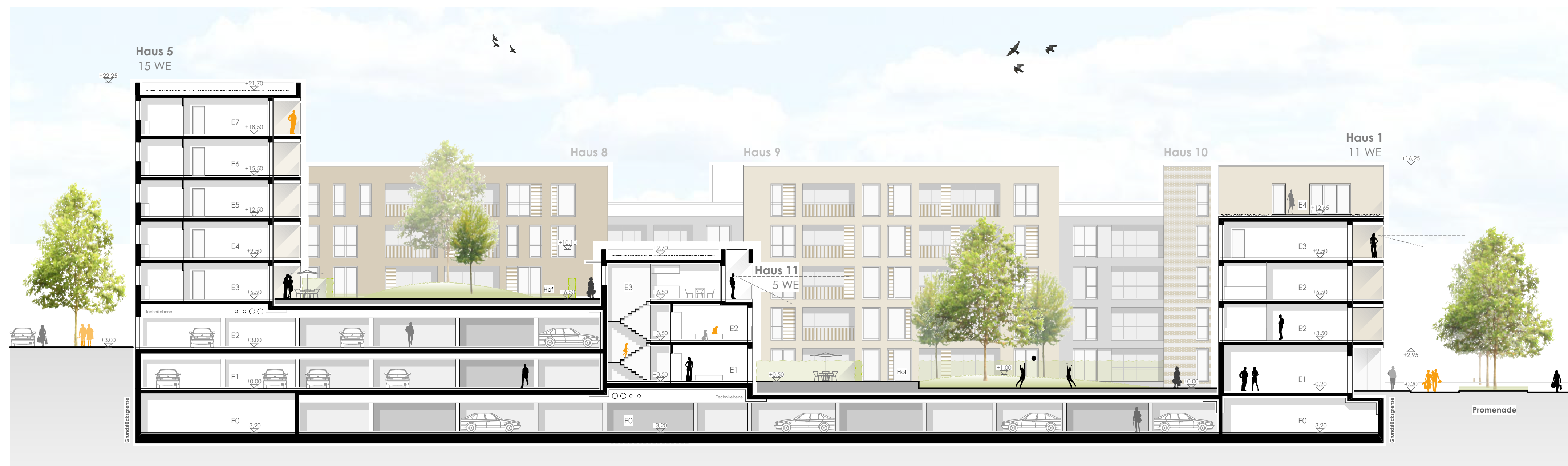
Schnitt B-B, M 1:200
