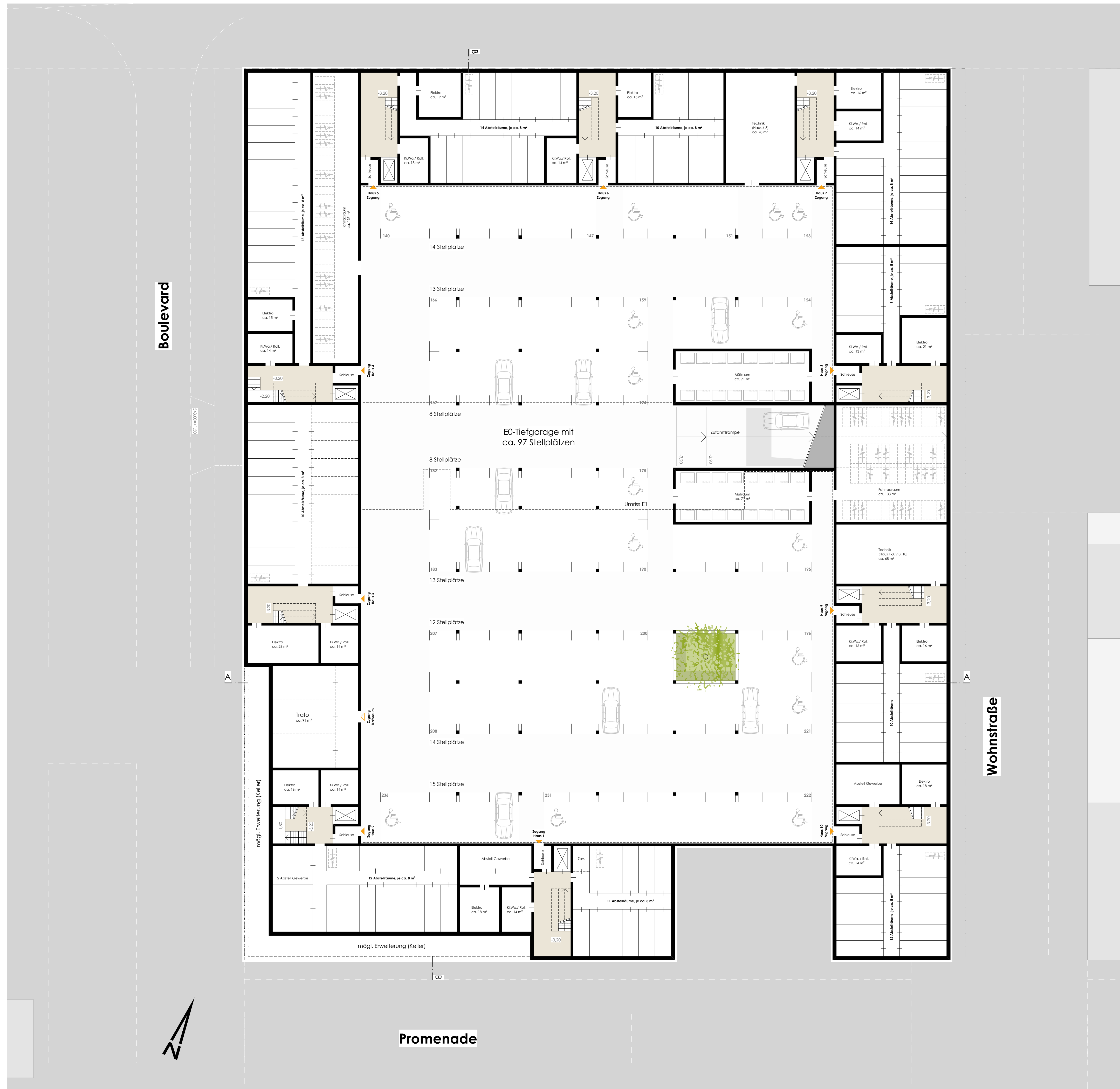
Ebene 0 (-3,20), M 1:200
