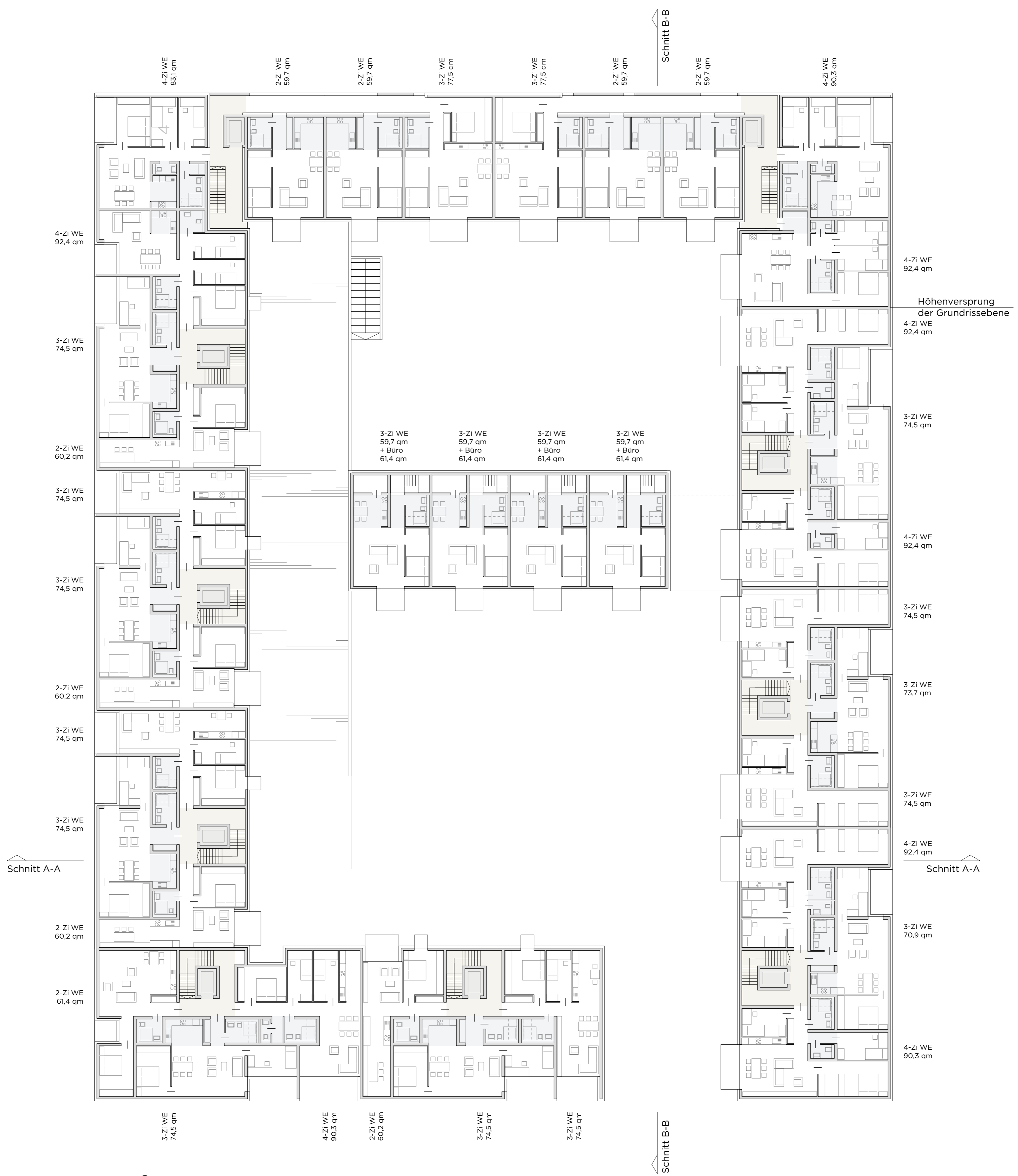
Grundriss 1. Obergeschoss | M 1:200
