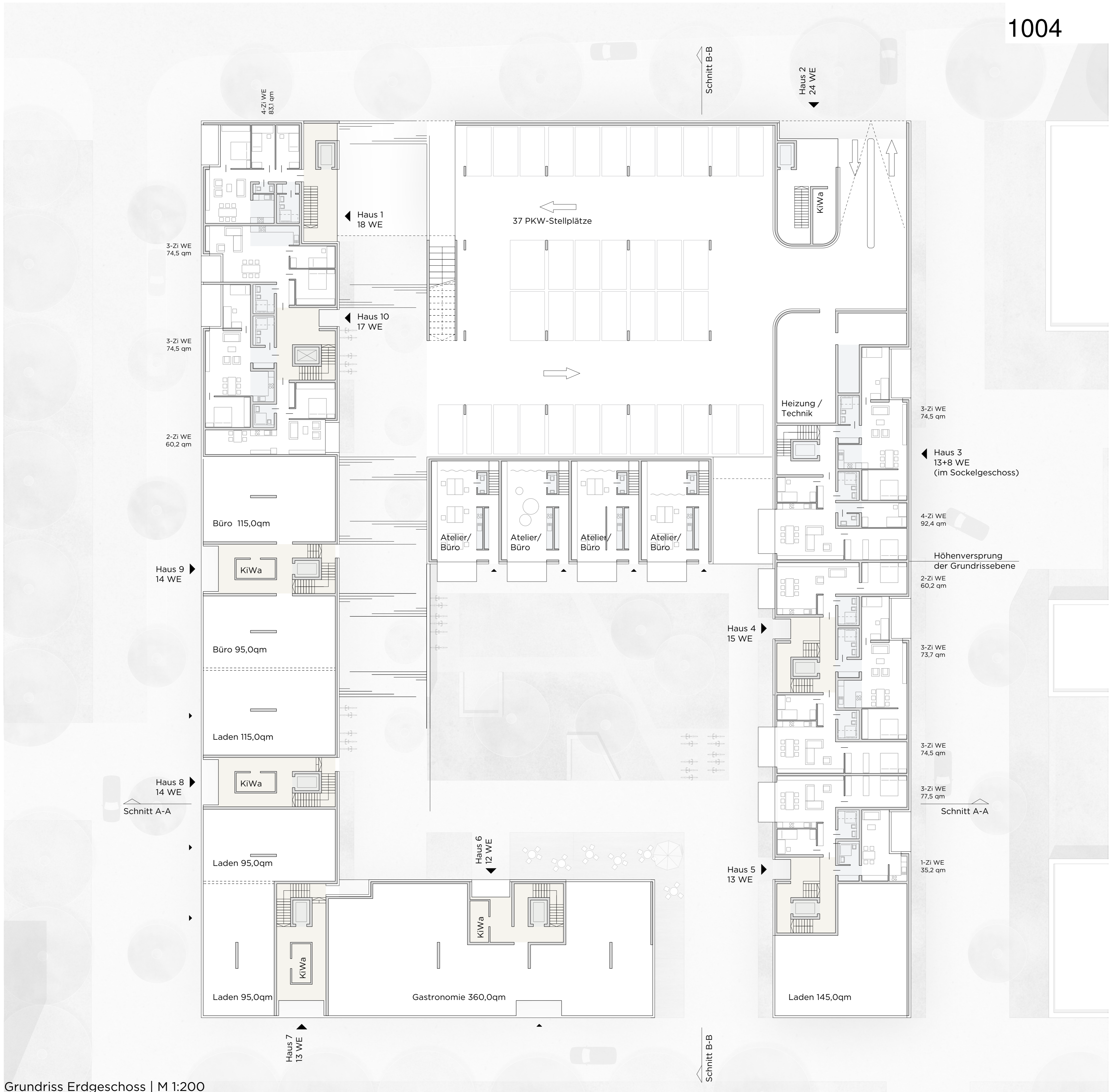
Grundriss Erdgeschoss | M 1:200
