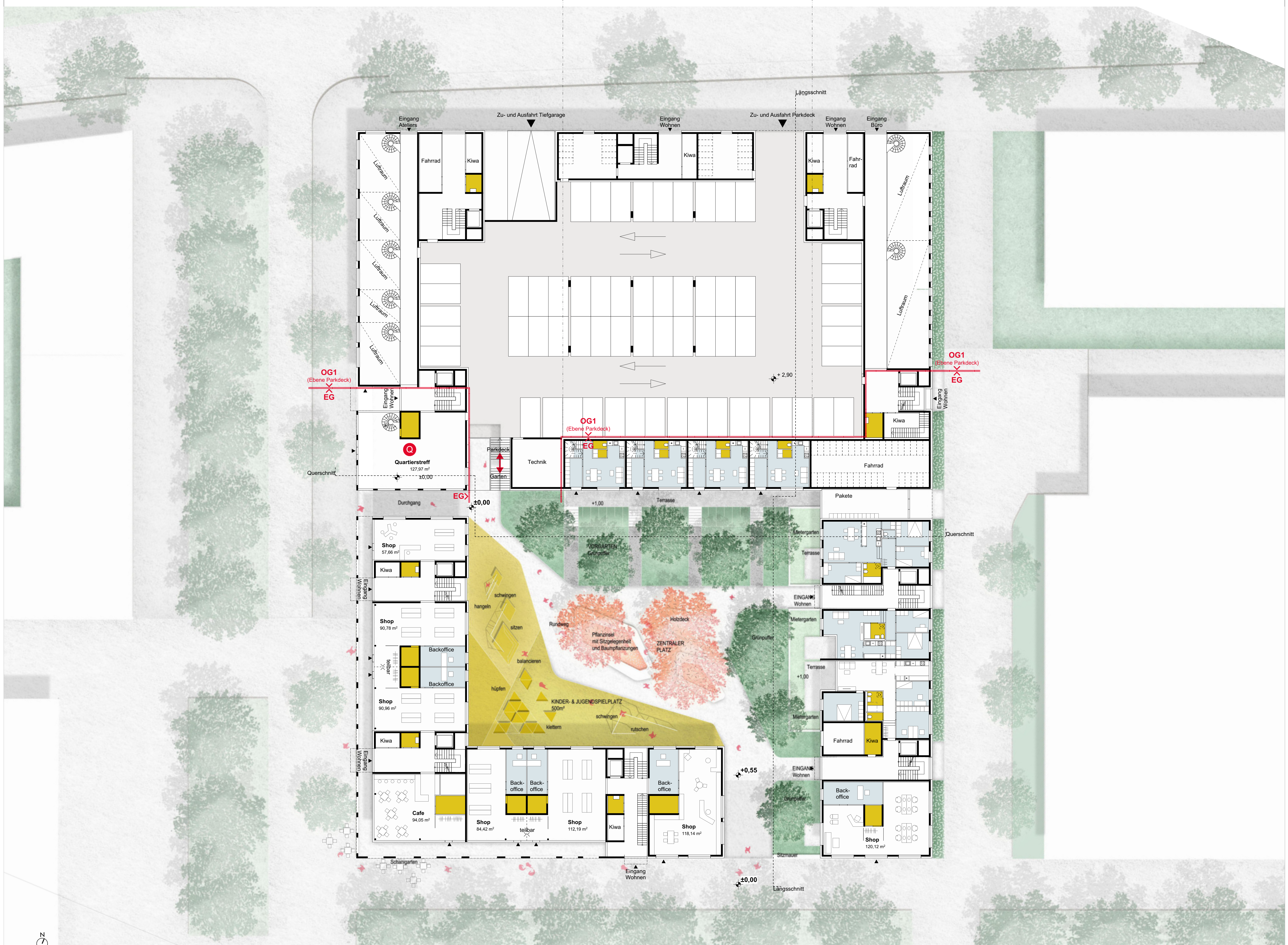
Grundriss EG-OG1 M 1:200
